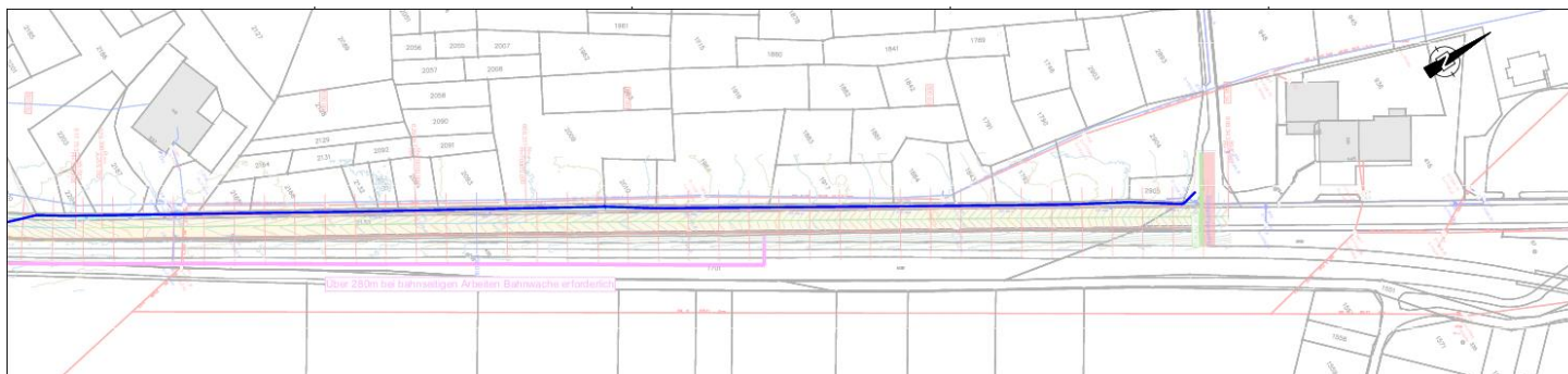
Plan Leitungsführung Reckingen-Münster
