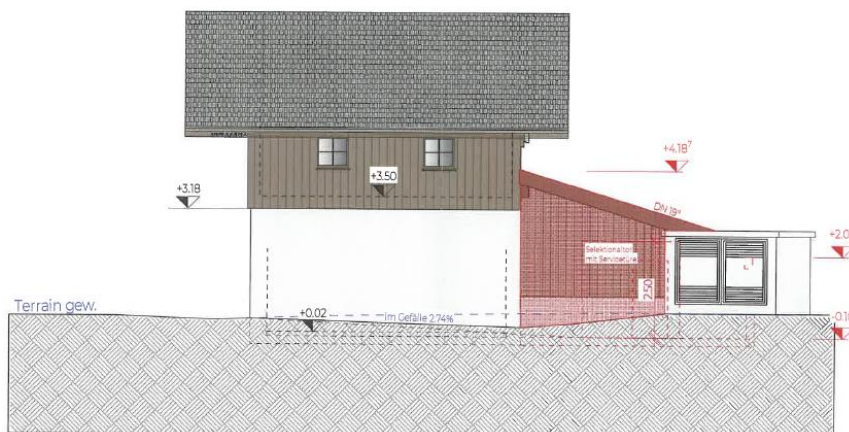
Ansicht West
